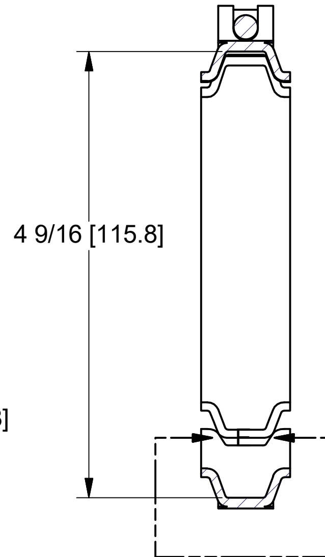
SECTION D-D SCALE 1 : 1
